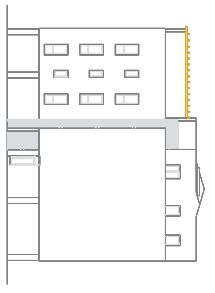
PIANTA ATTICO
